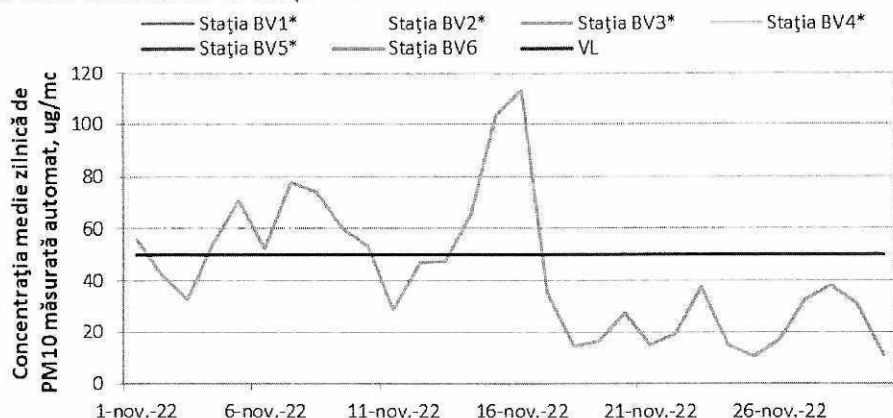
Figura 1.1.2.4.3. Evoluția mediilor zilnice de PM 10, metoda automată, în luna noiembrie
